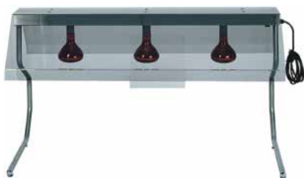
TELAIO CON LAMPADE INFRAROSSI DA APPENDERE STRUCTURE A MUR AVEC LAMPES A INFRAROUGES FRAME WITH INFRARED LAMPS TO BE HANGED GESTELL MIT INFRAROTLAMPEN UM ZU AUFHAENGEN
