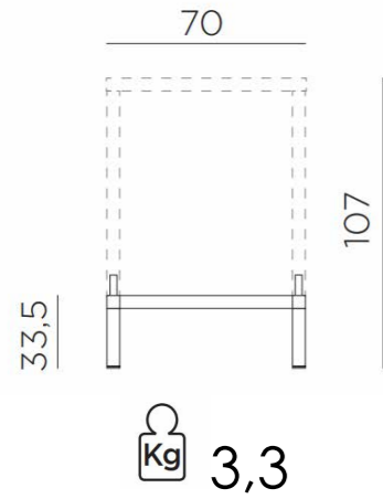
KIT PER CUBO 70
