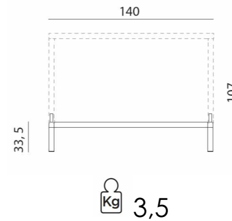
KIT PER CUBO 140X80
