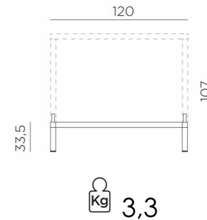
KIT PER CUBO 120X70
